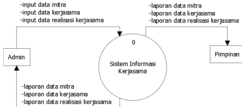
Gambar 3 Diagram konteks
