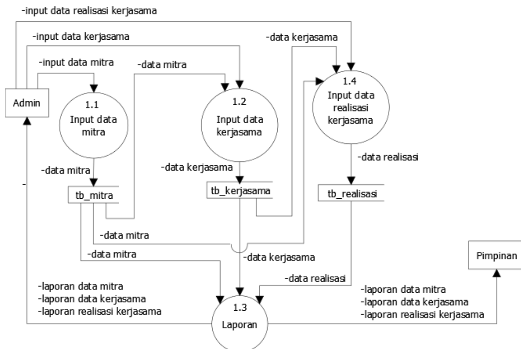
Gambar 4 DFD Level 1
